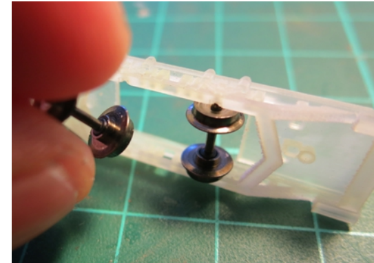
Montage (N1102)
